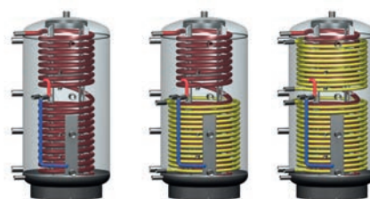
Systeembuffer met geïntegreerde inox warmtewisselaar, zonder of met 1 of 2 zonnewarmtewisselaars
