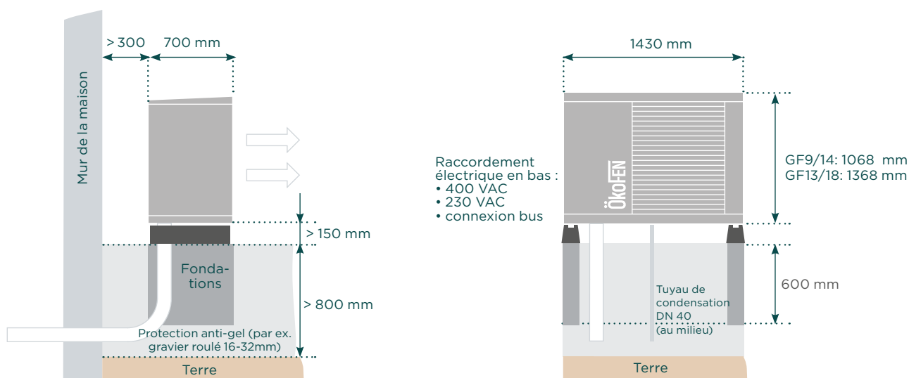
Schéma d'installation : Plan détaillé des fondations dans les documents de planification
